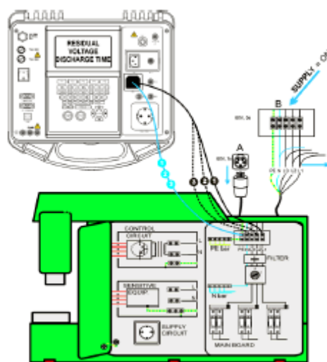
Prüfung der Entladezeit
