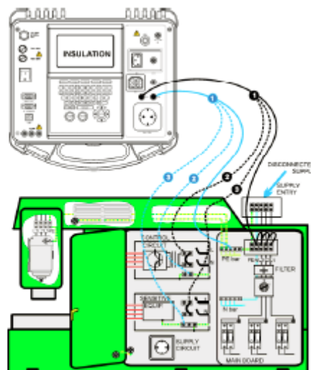
Messung des Isolationswiderstands
