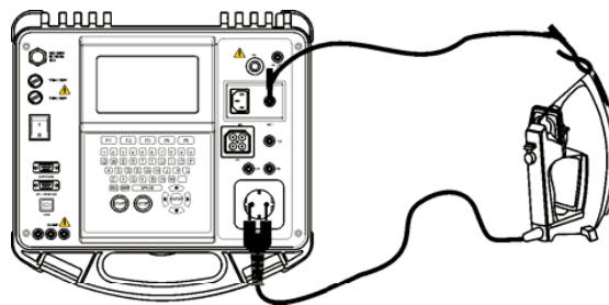
Messung des Schutzleiterwiderstands am Prüfling der Klasse 1.
