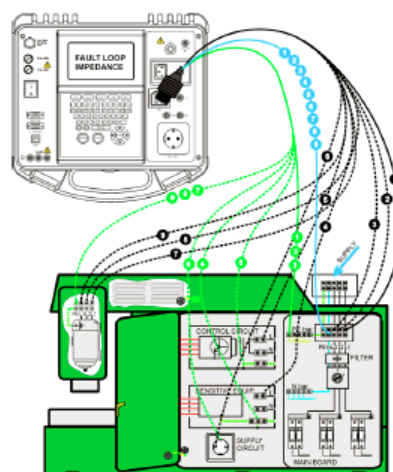
Messung der Fehlerschleifenimpedanz
