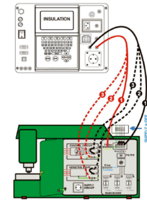
Messung des Isolationswiderstands
