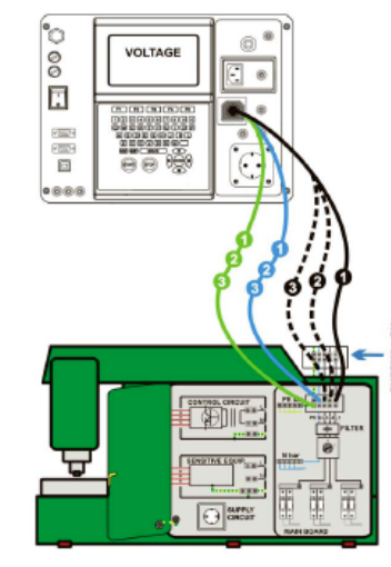
Spannungsprüfung
