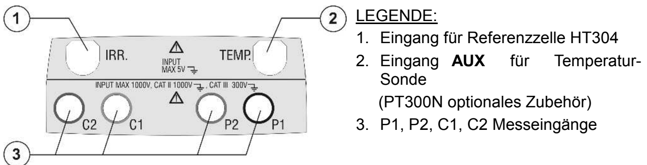
Abb. 3: Beschreibung Kopfteils vom Instrument
