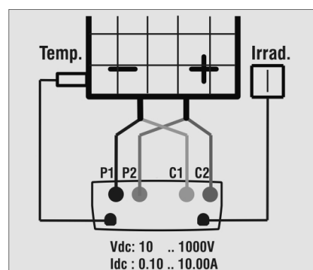
Abb. 1: Anschluss-Schema
